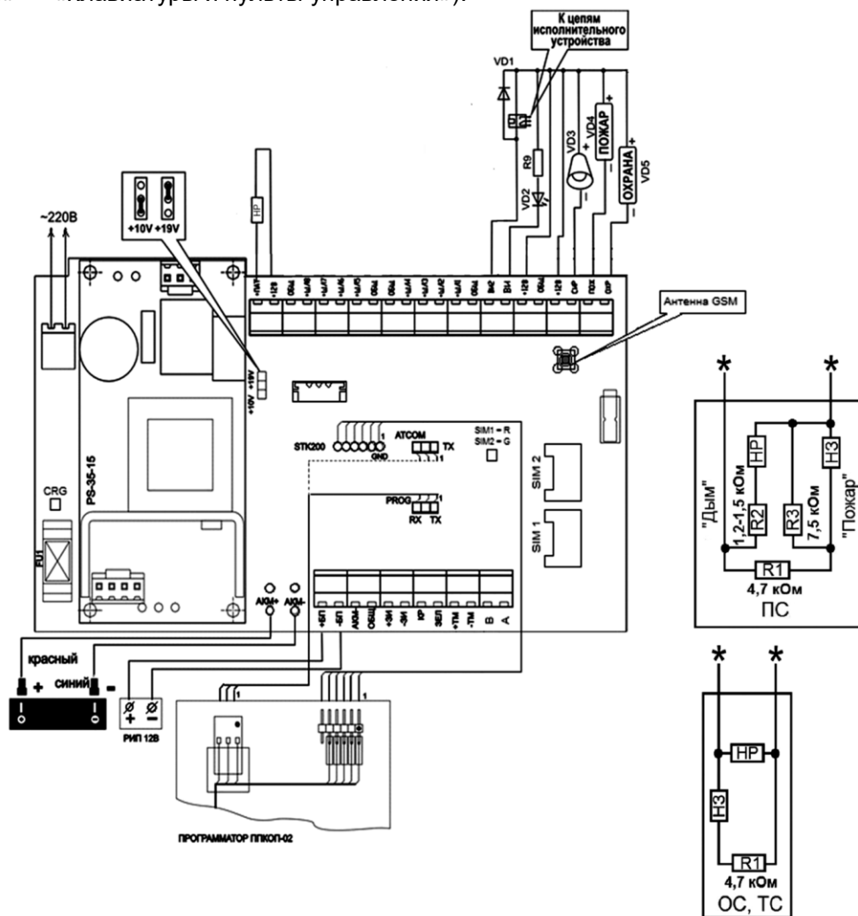
Рисунок 1. Схема подключения прибора
