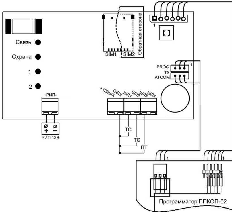
Рисунок 2 – Схема подключения ТК
