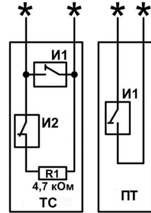
Рисунок 3 – Схема организации ШС
