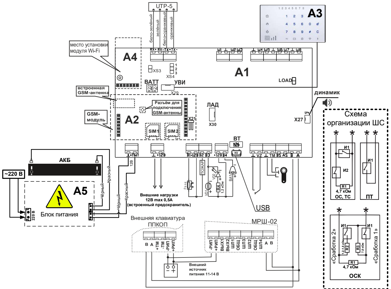
Рисунок 6 – Схема подключения прибора версии Приток-А-КОП-04
