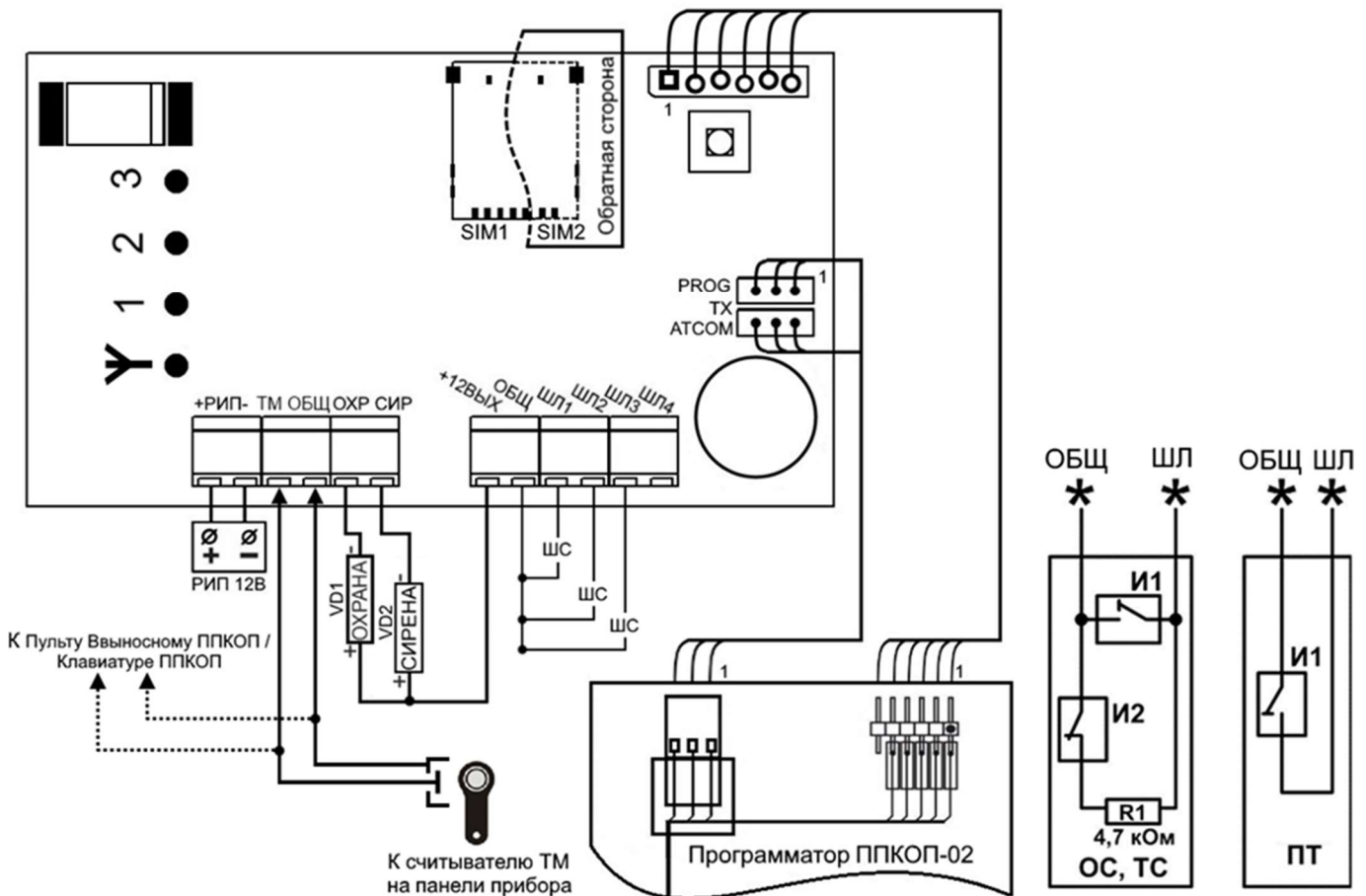
Рисунок 2 – Схема подключения прибора и организация ШС
